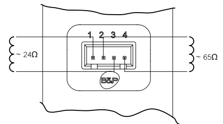
fig. 11 - Conexión de la válvula de gas
