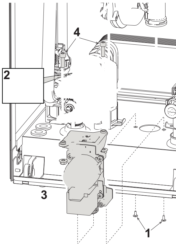
fig. 35- Sustitución de la válvula de gas
