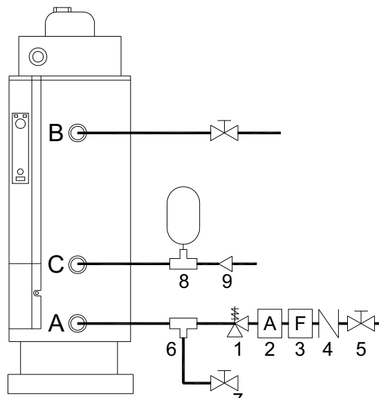
fig. 2.5/2 : connessioni mod. 150-180
