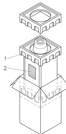
fig. 1.2/1 : imballo mod. 80 - 120
