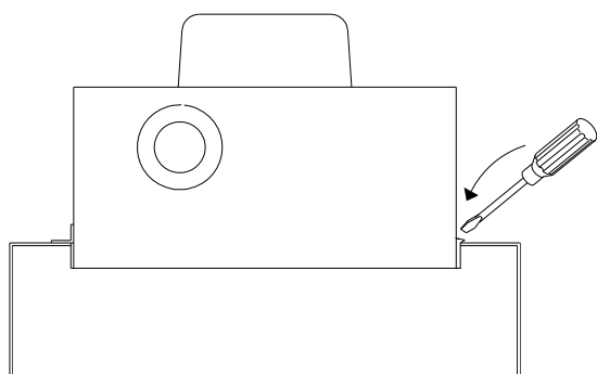
fig. 2.4/2 : inserzione guarnizione
