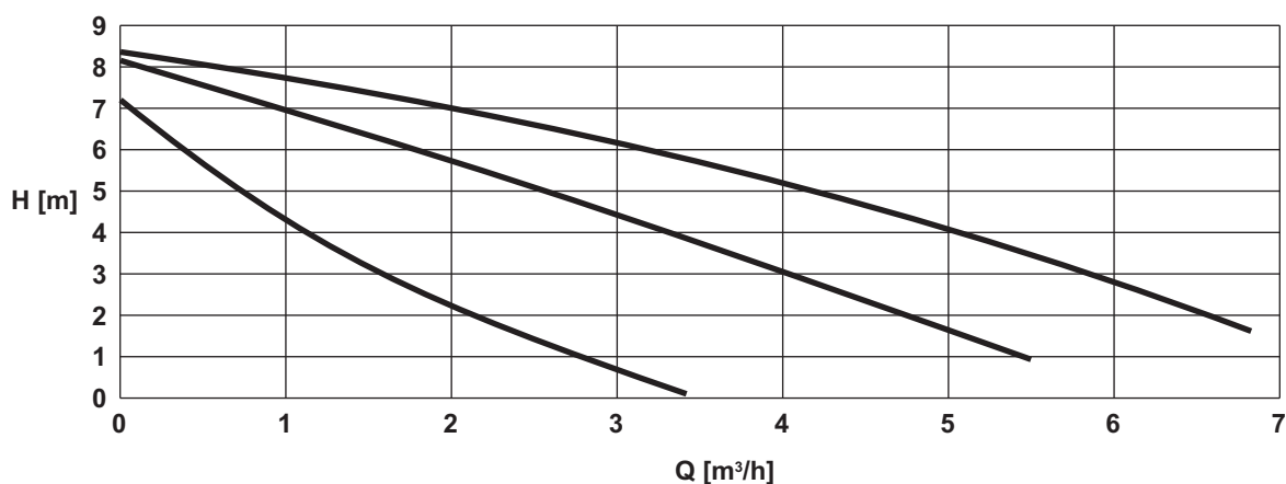
fig. 16 - Prevalenza pompa
