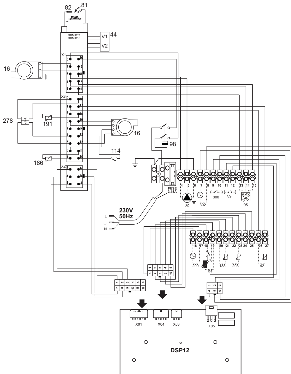
fig. 32 - Schema elettrico
