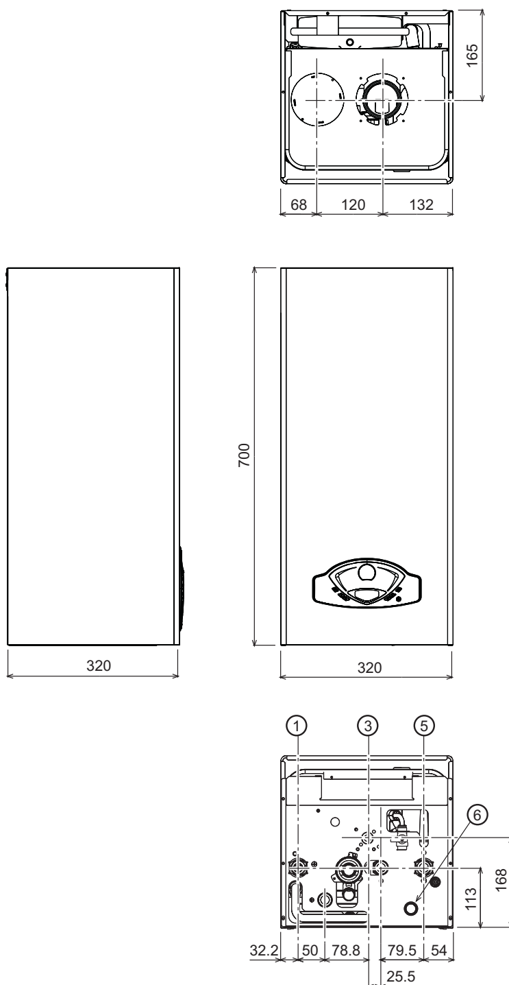
fig. 29 - Dimensioni e attacchi
