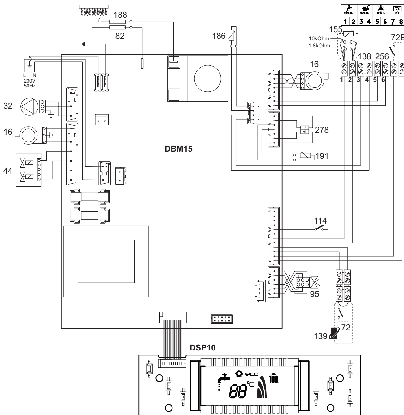
fig. 32 - Schema elettrico
