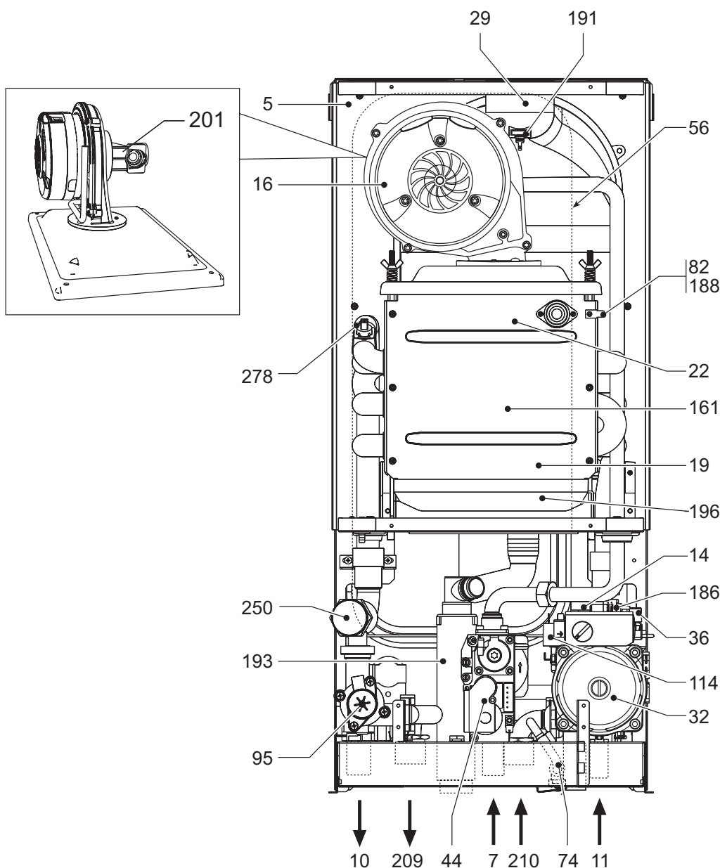
fig. 30 - Vista generale
