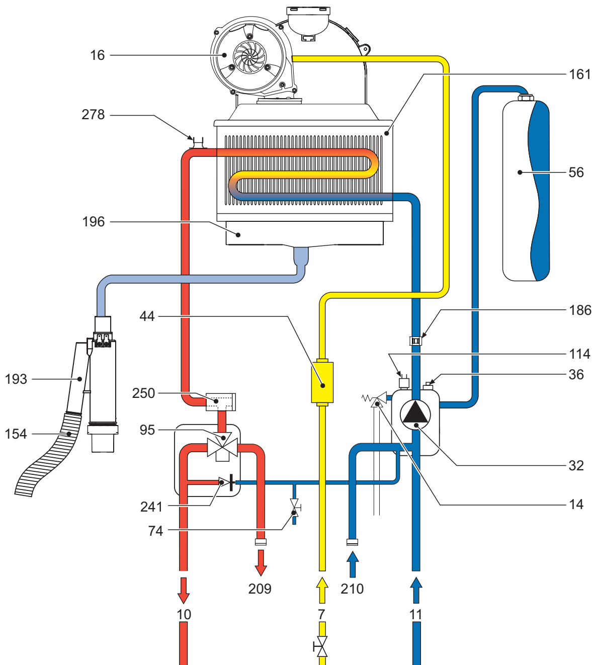
fig. 31 - Circuito idraulico
