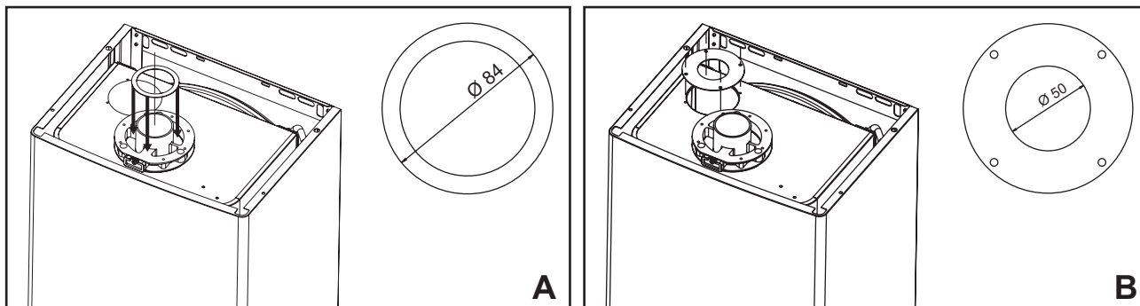
fig. 20 - Sustitución del diafragma
