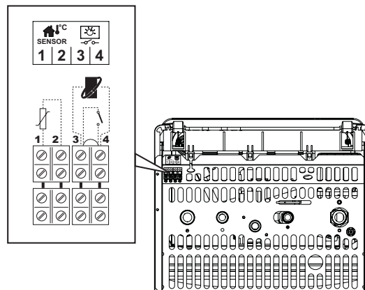
fig. 19 - Acceso a la regleta de conexiones
