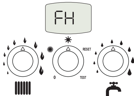
fig. 6 - Accensione caldaia
