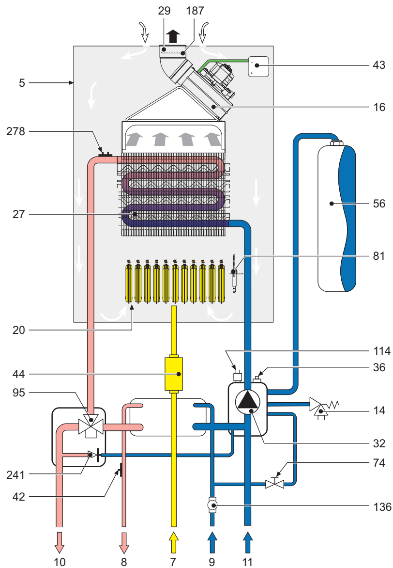
fig. 25 - Circuito idraulico
