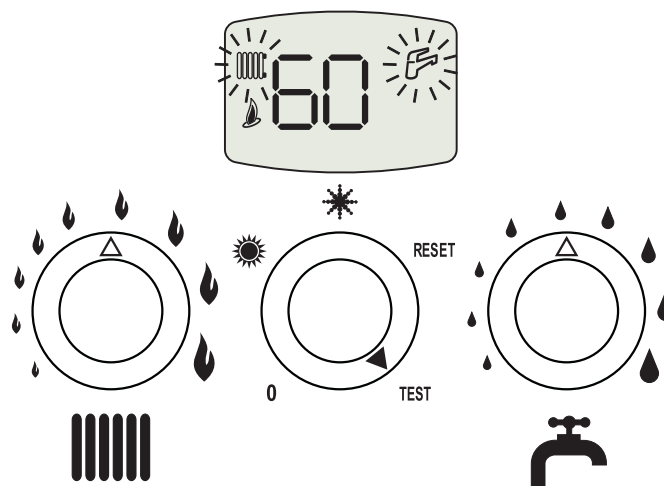
fig. 20 - Modalidad TEST (potencia de la calefacción = 100%)
