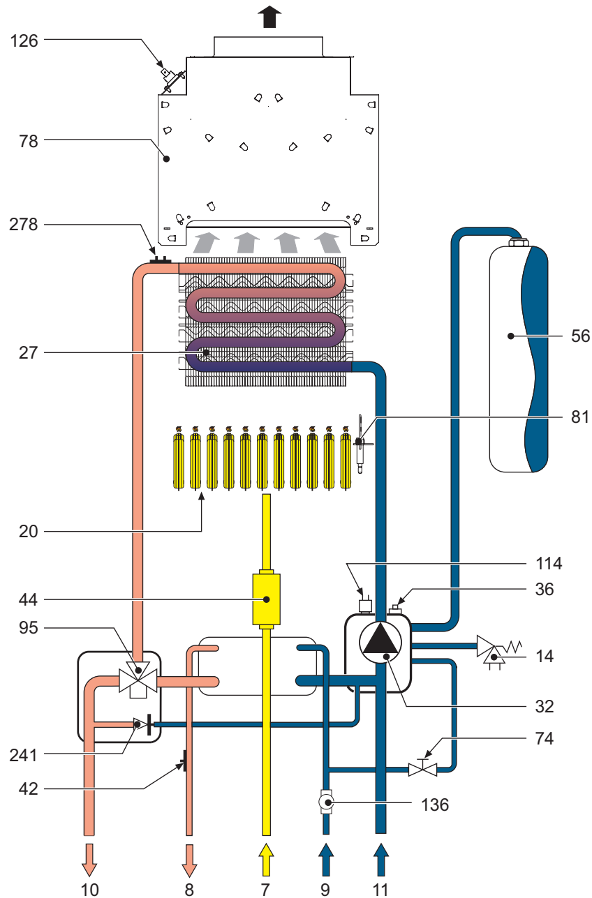
fig. 25 - Circuito hidráulico
