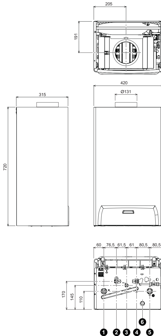
fig. 23 - Dimensiones y conexiones
