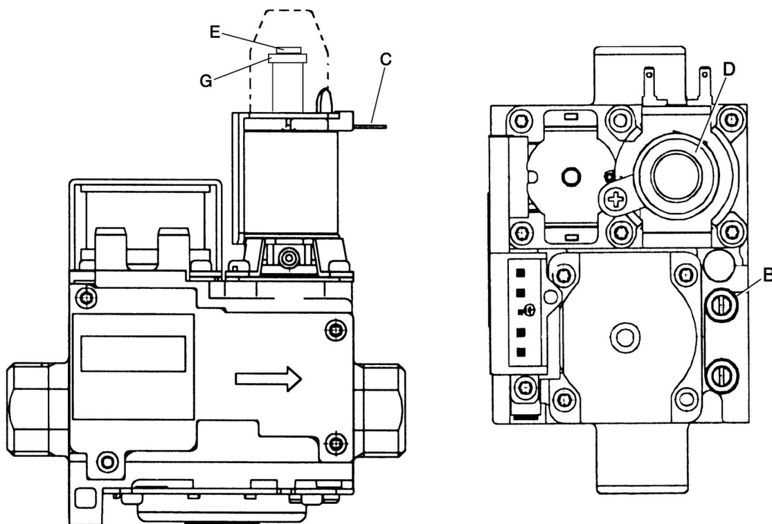
fig. 21 - Válvula de gas
