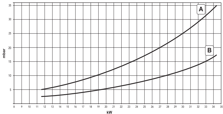
fig. 18 - Diagrama presión - potencia (TAURA D 32 MCA)
