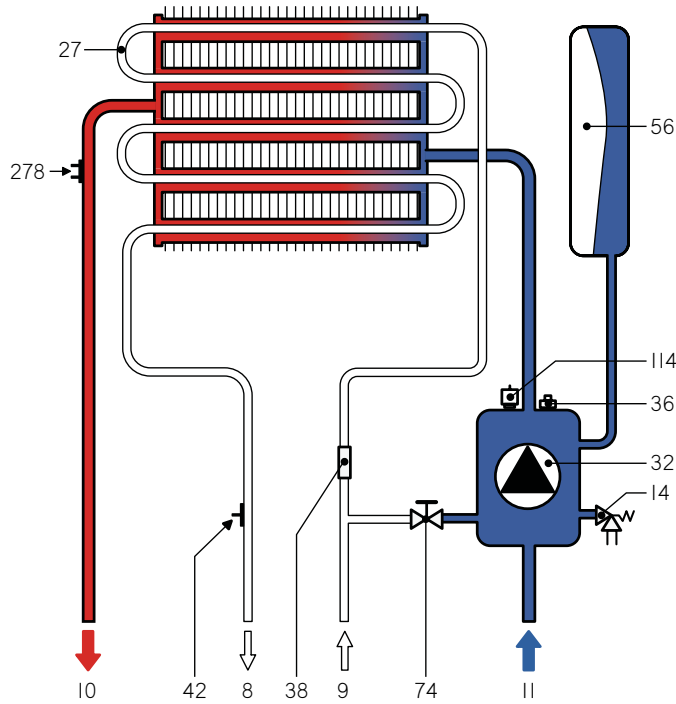
fig. 15 - Circuito de calefacción
