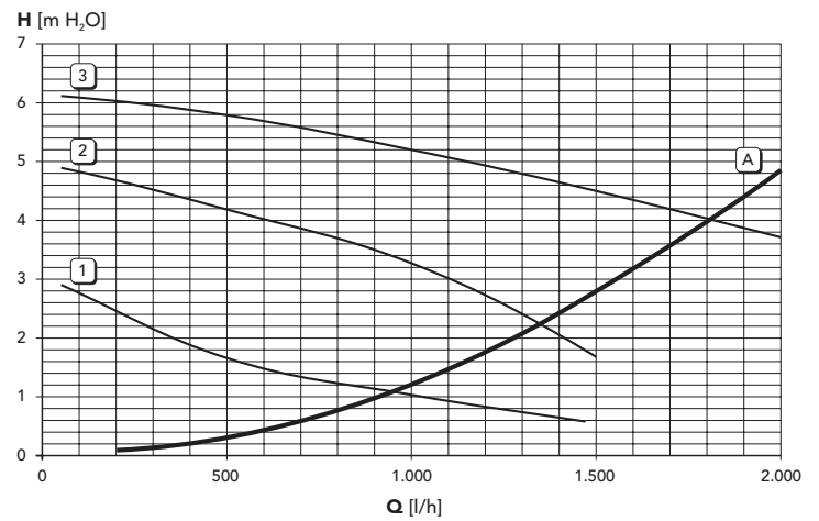
fig. 20 - Pérdidas de carga / altura manométrica bombas de circulación (TAURA D 32 MCA)
