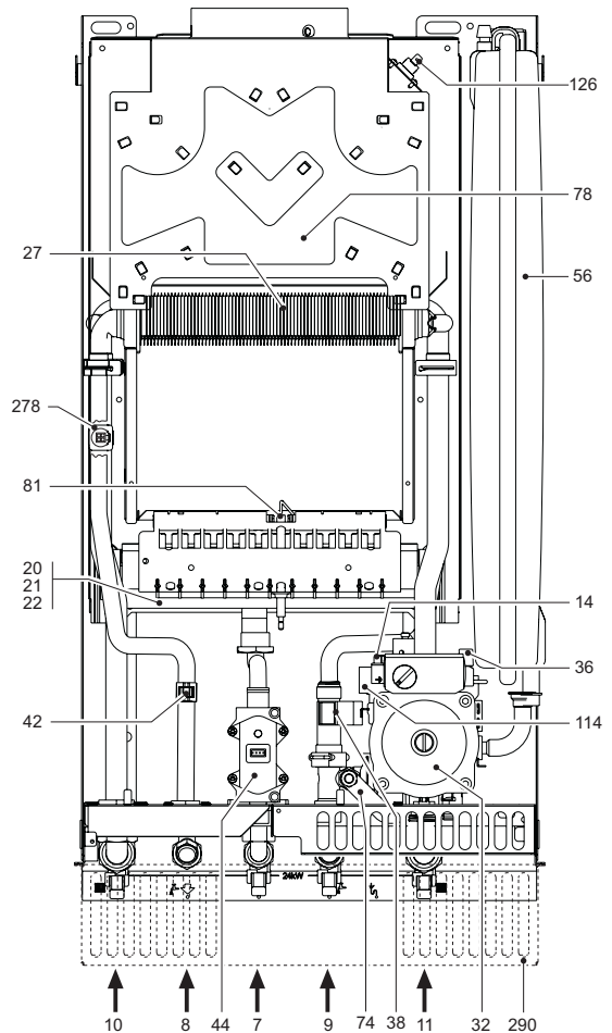
fig. 13 - Vista general TAURA D 24 MCA
