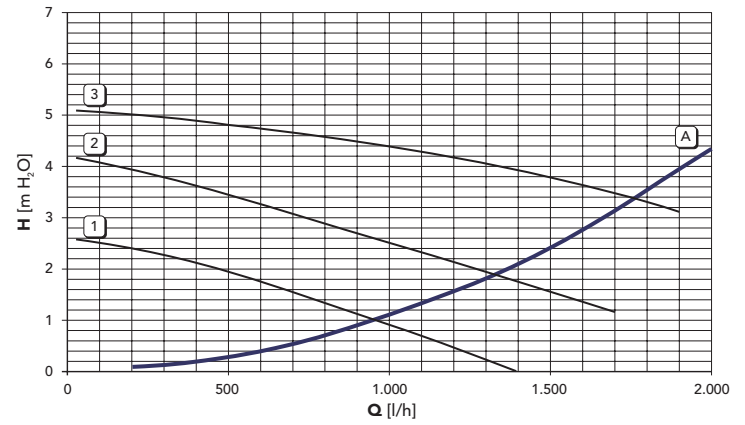
fig. 19 - Pérdidas de carga / altura manométrica bombas de circulación (TAURA D 24 MCA)
