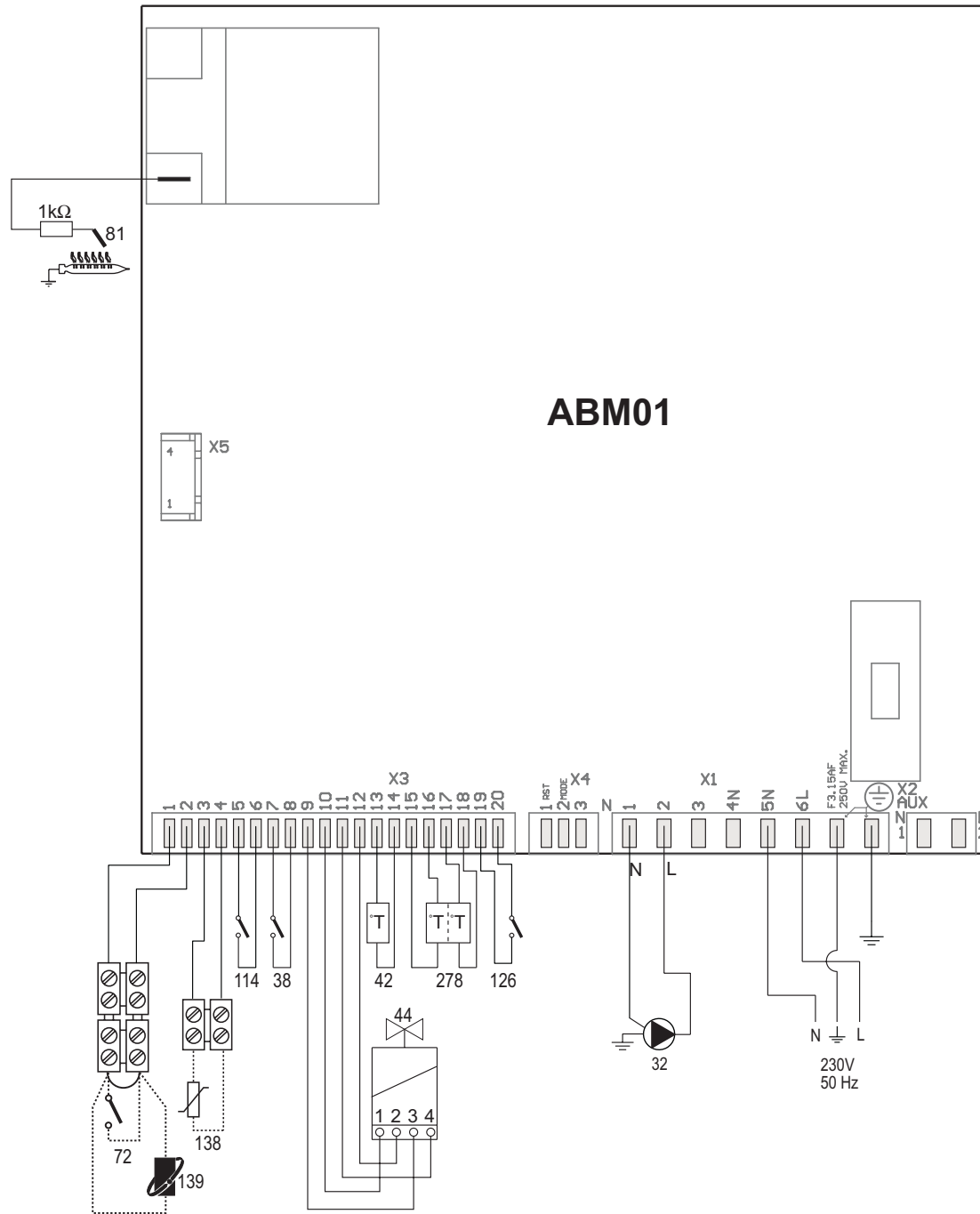
fig. 21 - Circuito eléctrico
