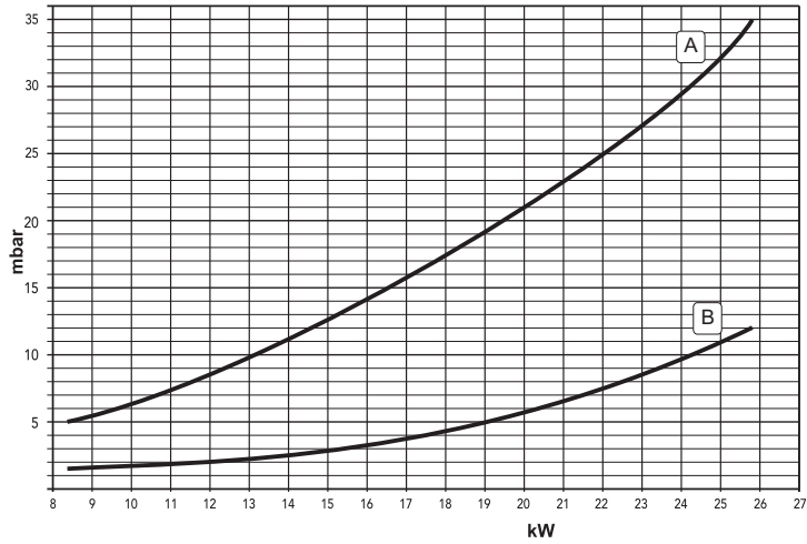
fig. 17 - Diagrama presión - potencia (TAURA D 24 MCA)
