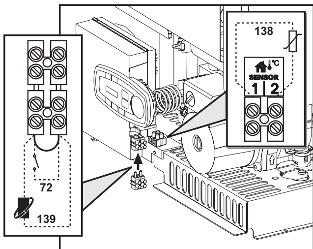
fig. 8 - Acceso a la regleta eléctrica
