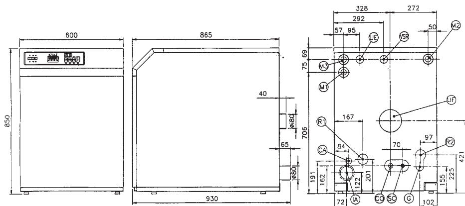
Fig. 1 - Dimensioni ed attacchi
