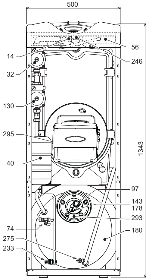
fig. 21 - Vista frontal
