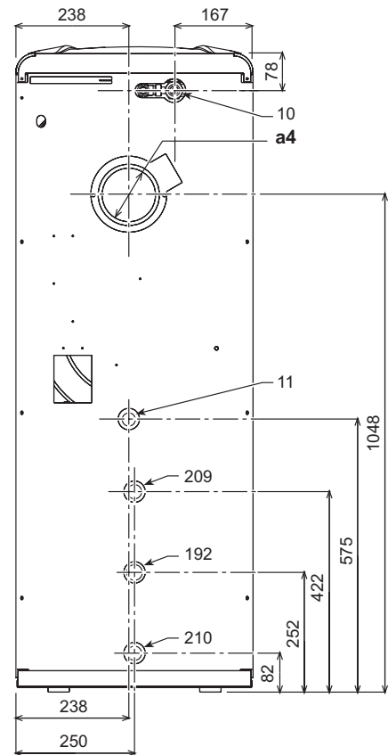
fig. 23 - Vista posterior
