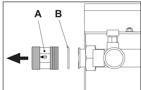
fig. 17 - Montaje de la válvula antirretorno
