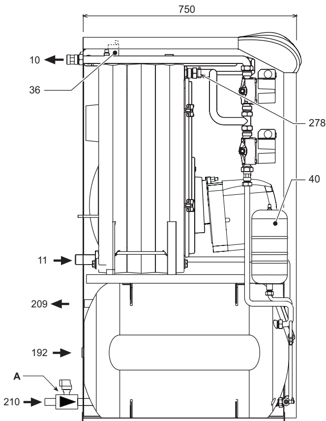
fig. 22 - Vista lateral
