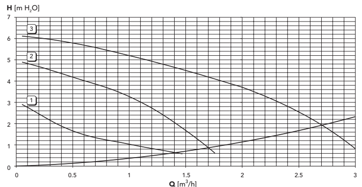
fig. 24 - Pérdidas de carga
