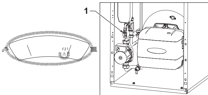
fig. 15 - Anomalía por baja presión en la instalación - Llave de llenado
