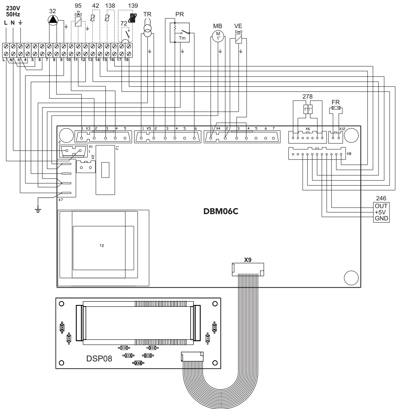
fig. 23 - Esquema eléctrico
