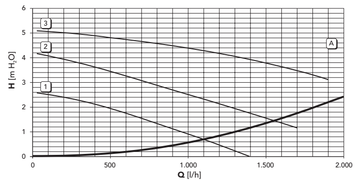
fig. 22 - Pérdida de carga / altura manométrica bomba
