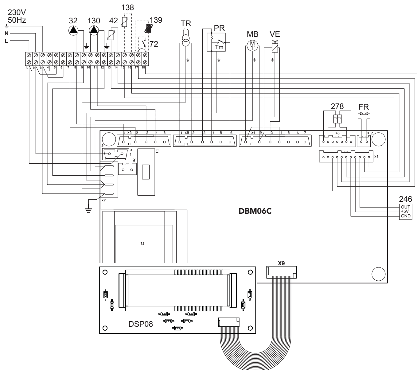
fig. 25 - Esquema eléctrico
