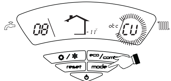
fig. 11 - Curva de compensación
