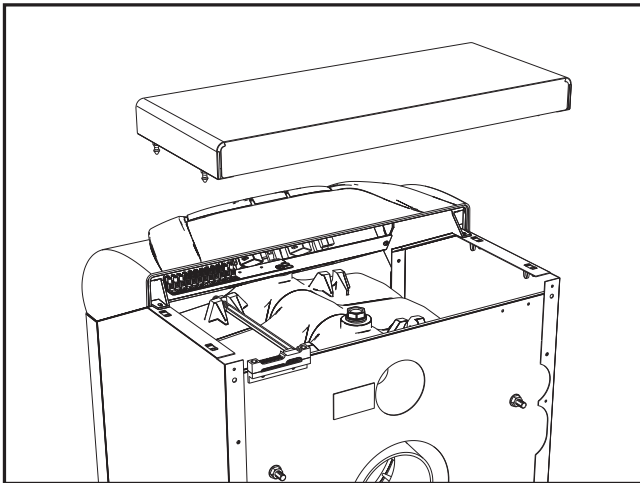
fig. 18 - Acceso a la regleta eléctrica
