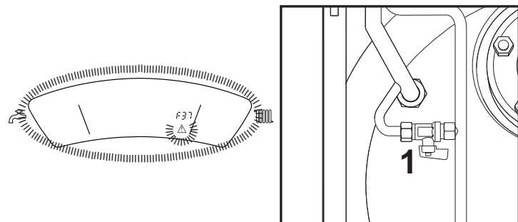
fig. 15 - Anomalía por baja presión en la instalación - Llave de llenado
