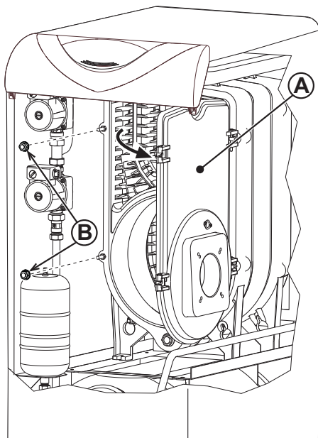
fig. 20 - Limpieza de la caldera
