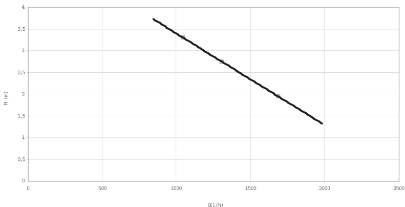
Altura manométrica disponible en los racores
