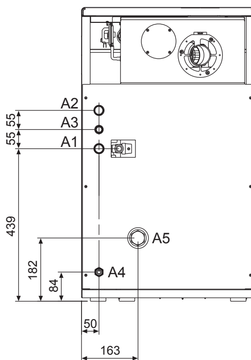
Vista posteriore mod. ERA F 32 SPK
