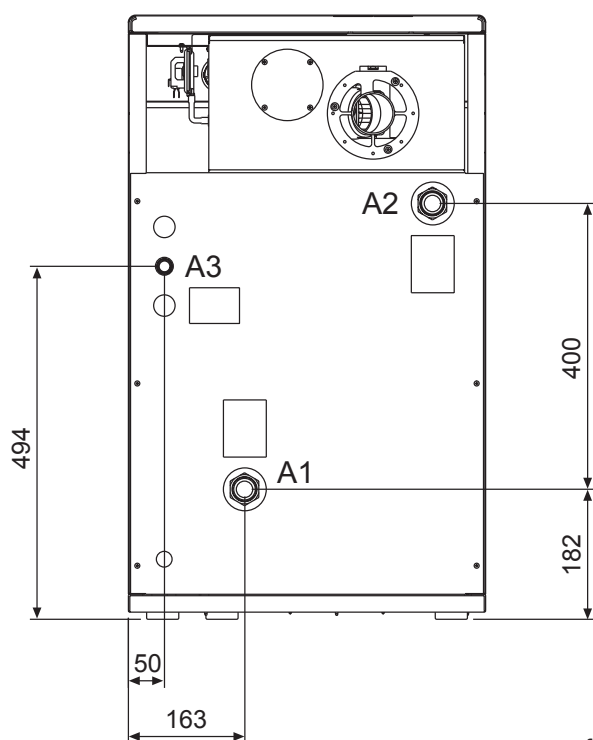
Vista posteriore mod. ERA F 32 S
