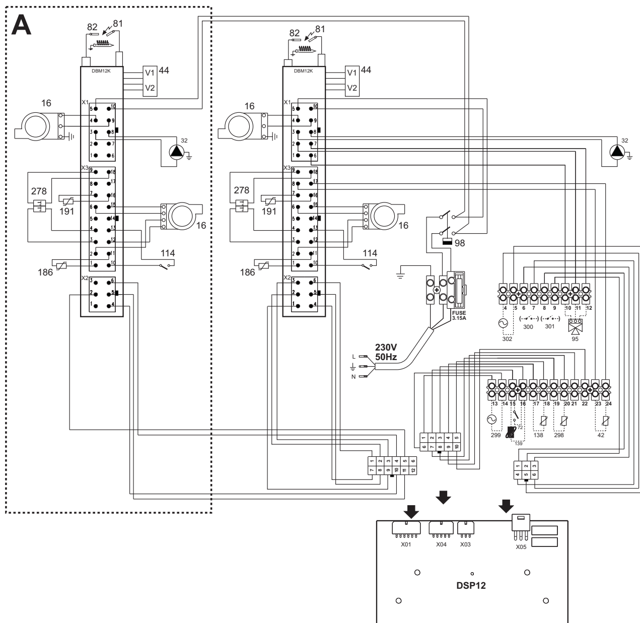
fig. 39 - Schema elettrico
